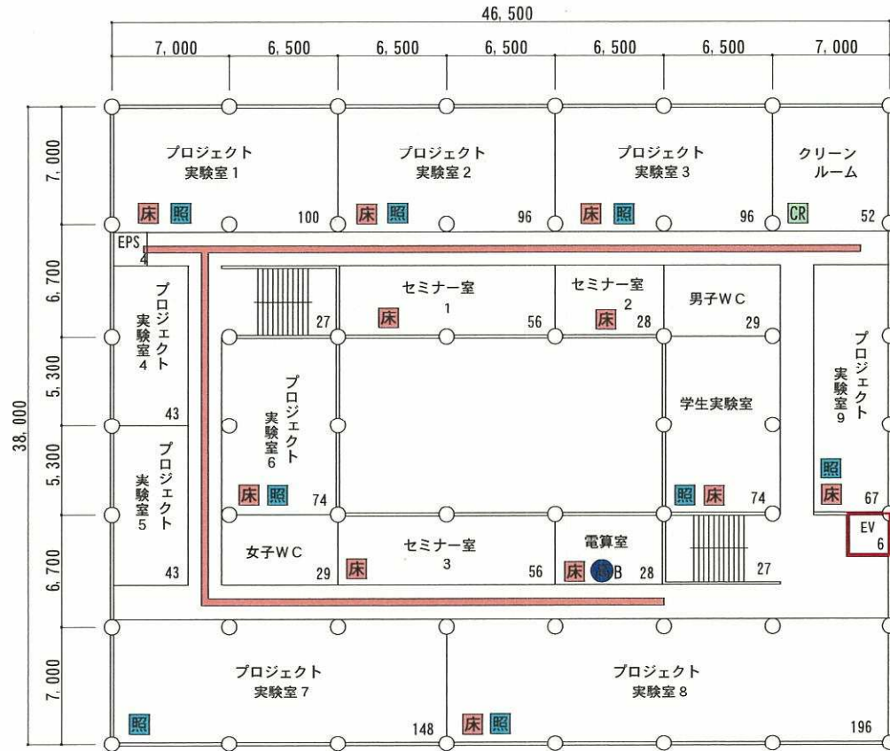
4階平面図
