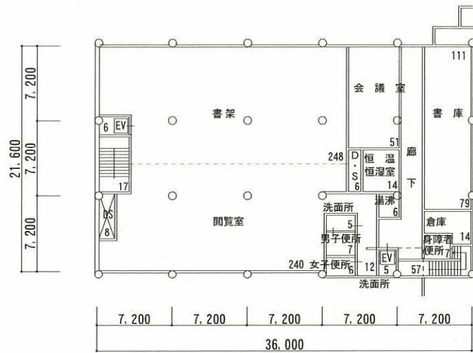
改修前 1階平面図
