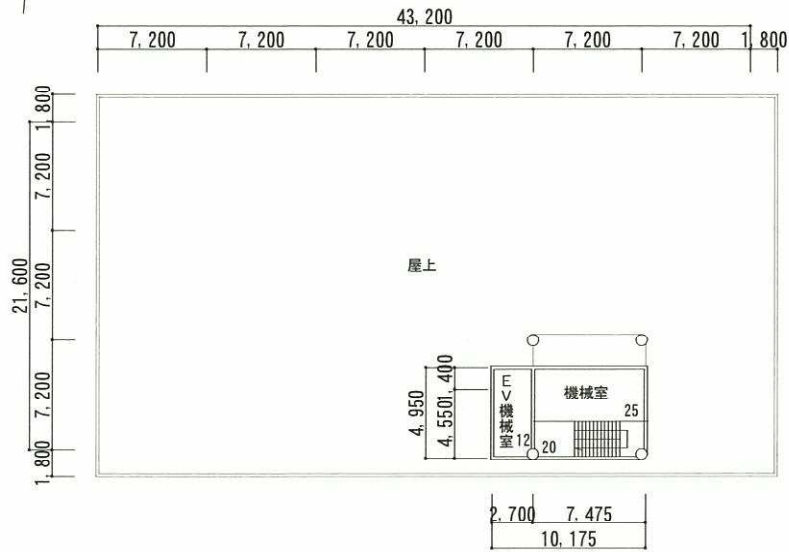
改修前PH階平面図
