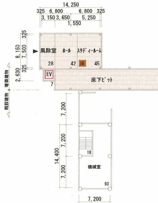
増築後地階平面図
