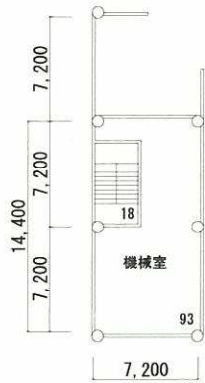
既設地階平面図
