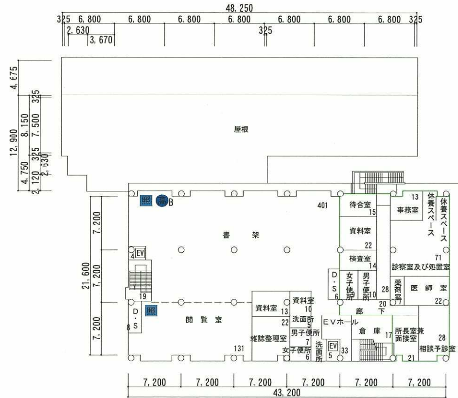
改修後3階平面図
