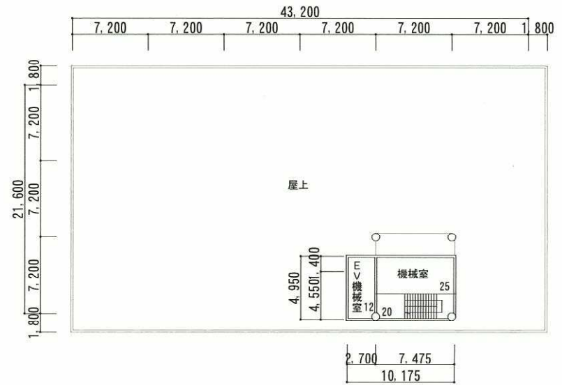
改修後PH階平面図
