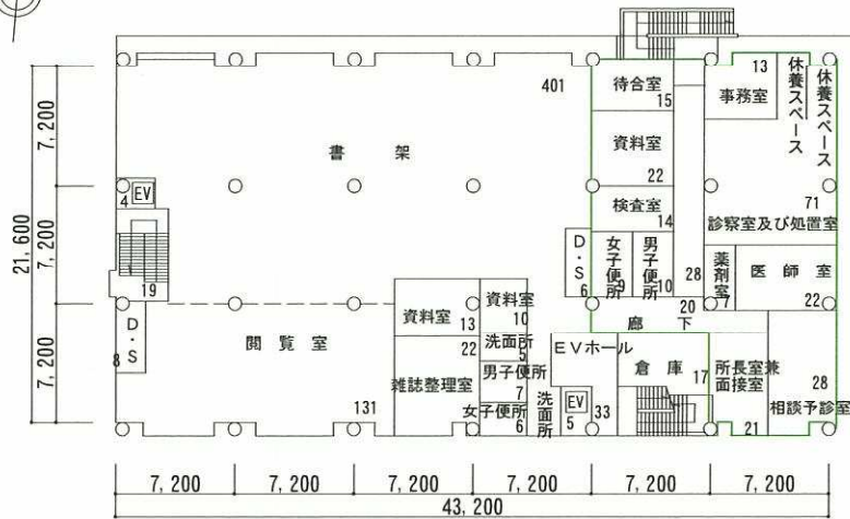
改修前3階平面図
