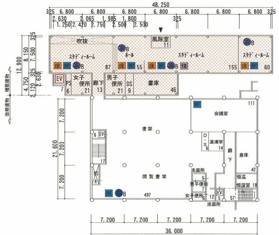
改修後 1階平面図
