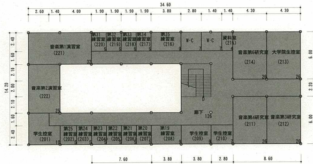
既設 2 階 平面 図
