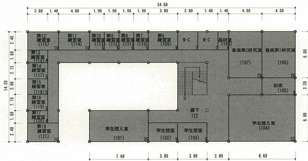
既設 1 階平面図
