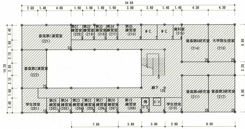
改修 2 階 平面 図
