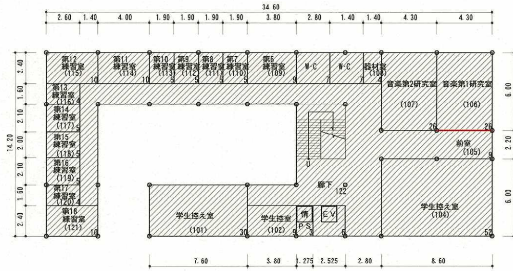
改修 1 階平面図
