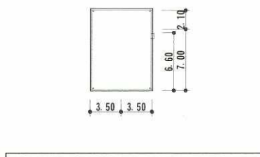
既設 P H 階平面図
