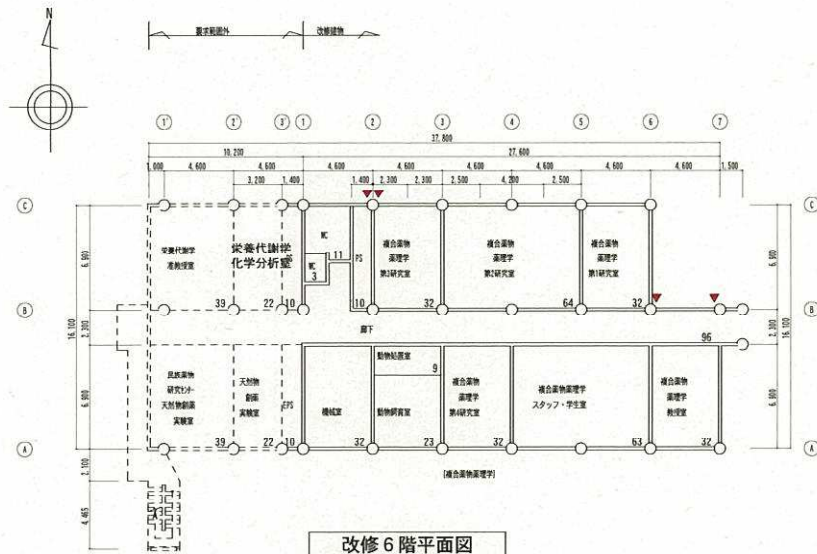
改修 6 階平面図
