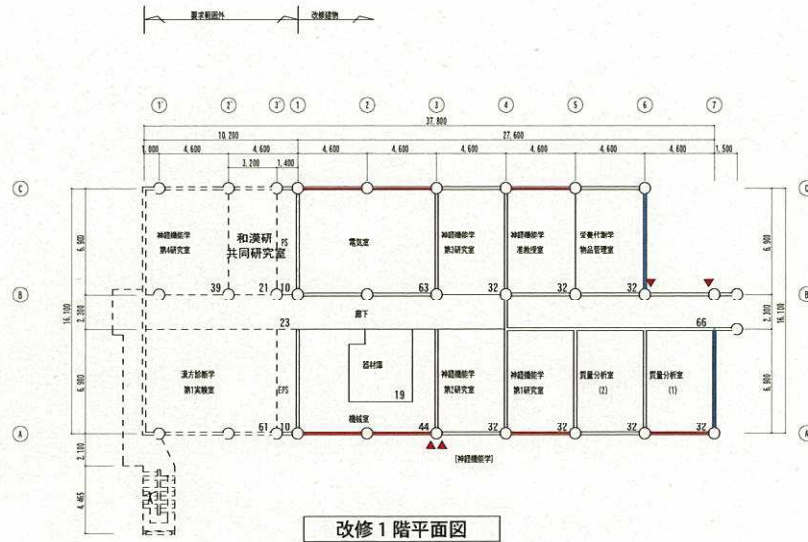
改修1階平面図
