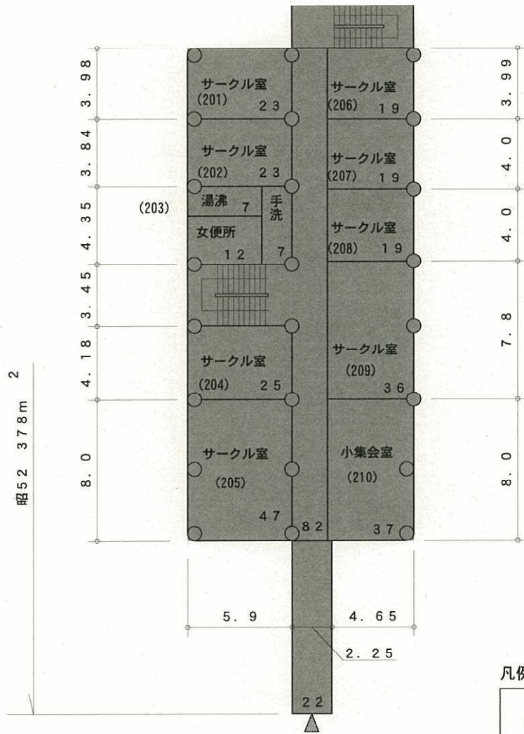
既設 2 階 平面図
