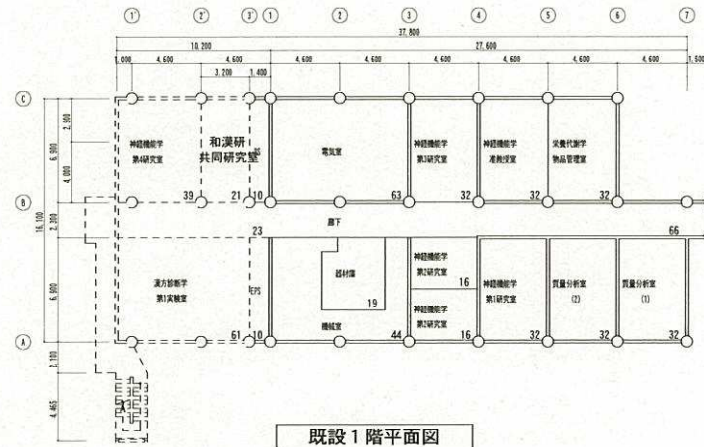
既設1階平面図
