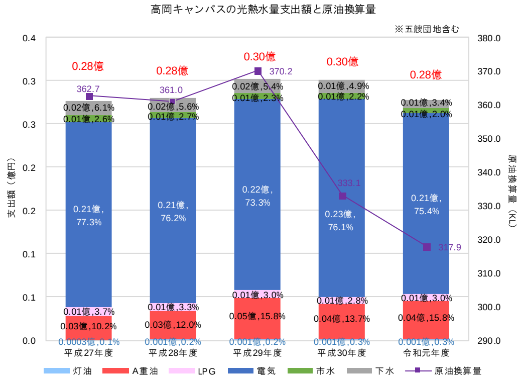
＜STEP1＞高岡キャンパスの光熱水量支出額と原油換算量
