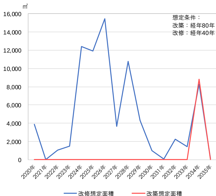
図表－R16 Mid-Term（2035年，令和17年）までの施設整備の需要の試算
