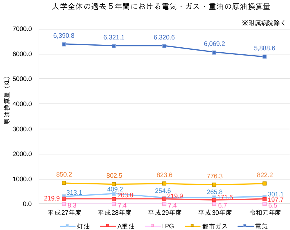
＜STEP1＞大学全体の過去5年間における電気・ガス・重油の原油換算量
