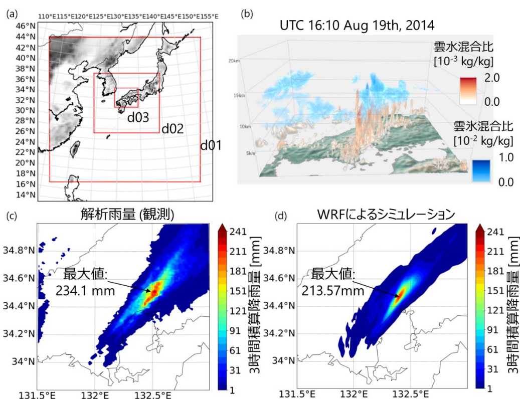
図 1. 気象モデル WRF を用いた 2014 年広島線の線状降水帯の再現計算。
