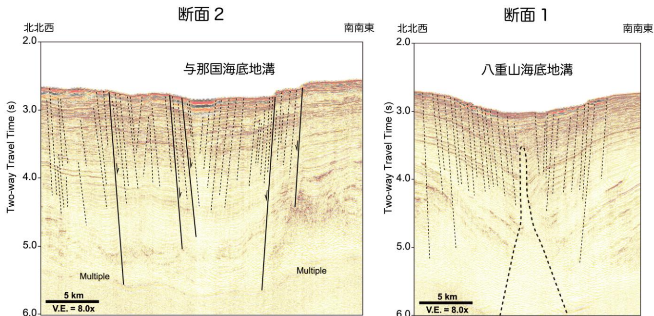
図 2 本研究で実施した反射法地震波探査による 2 つの海底地溝での正断層を含む地下構造 矢印は正断層の運動による沈下方向、実線と点線はどちらも正断層の面をそれぞれ示す。実線の正断層は点線の正断層よりも正断層運動による沈下量が大きい。
