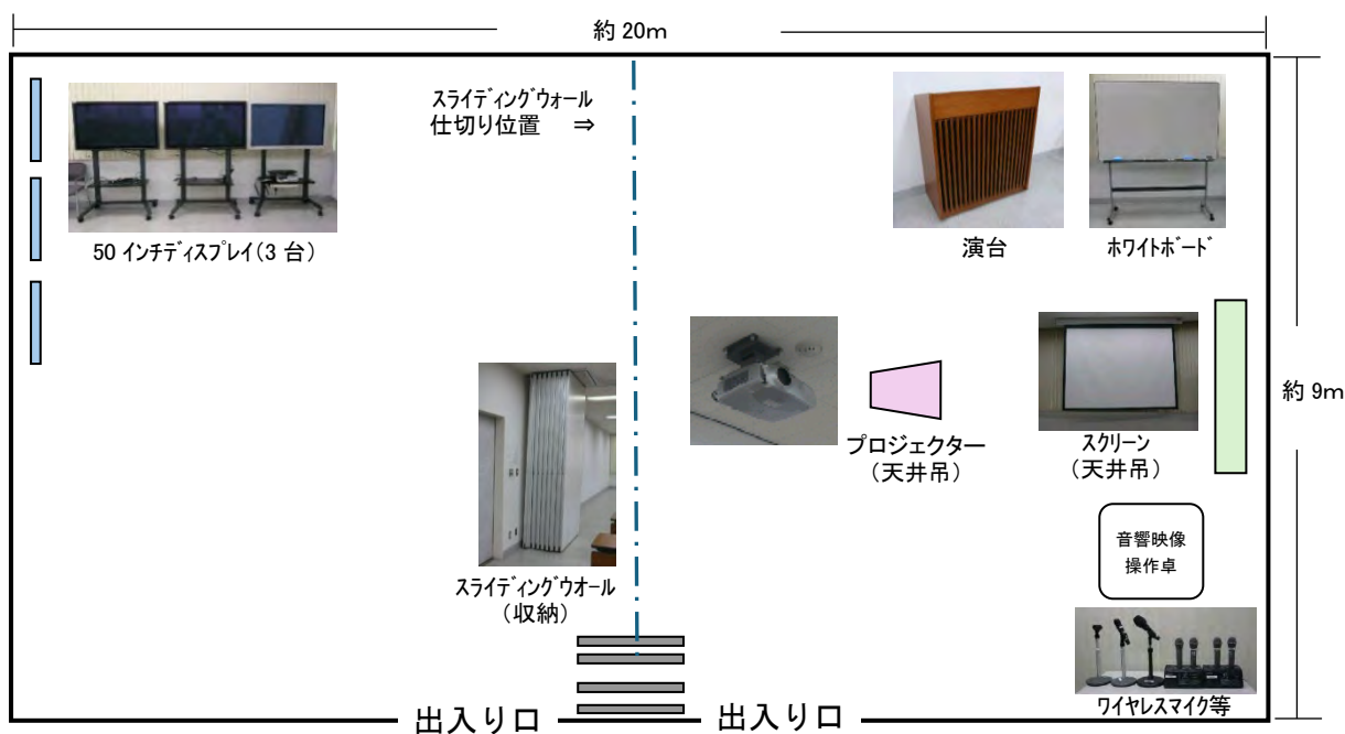
会議室平面図及び設備位置図
